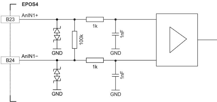
図 3-49 AnIN1 回路（AnIN2 も同様）
