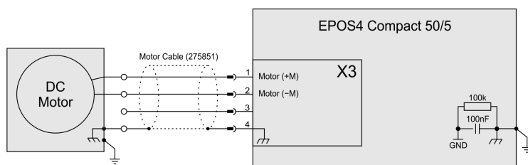
図 5-63 DC モータ
