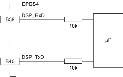
図 3-51 SCI 回路
