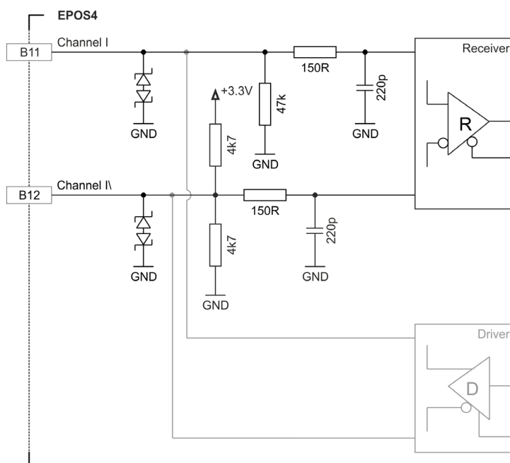
図 3-35 アナログ・インクリメンタル・エンコーダ入力回路 Ch I
