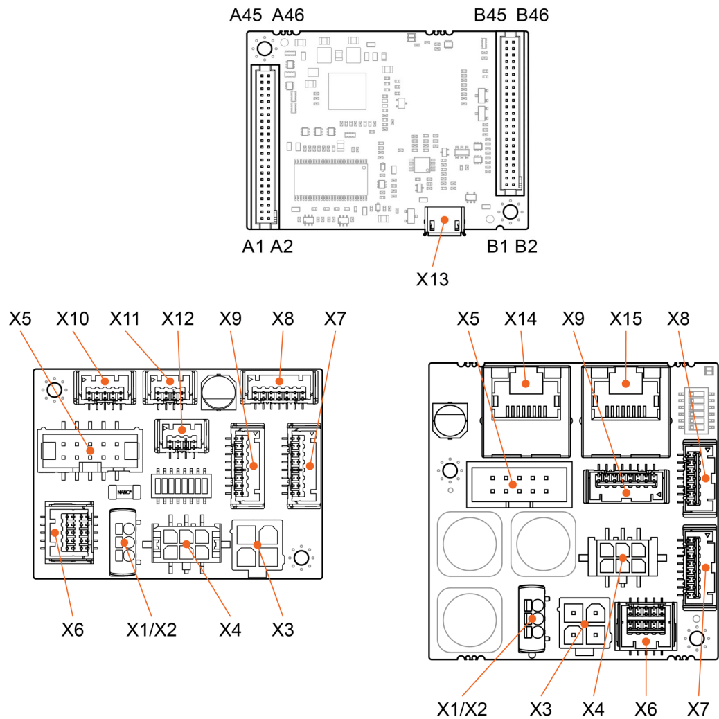
図 5-59 インターフェイス - 名称と取り付け位置
