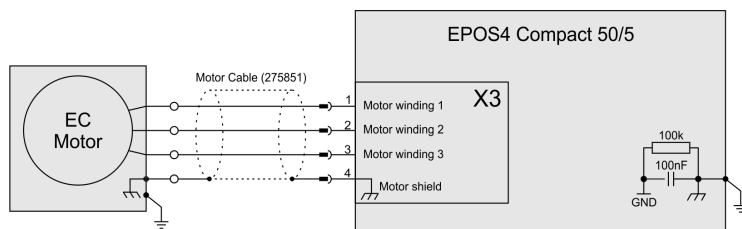
図 5-64 EC (BLDC) モータ
