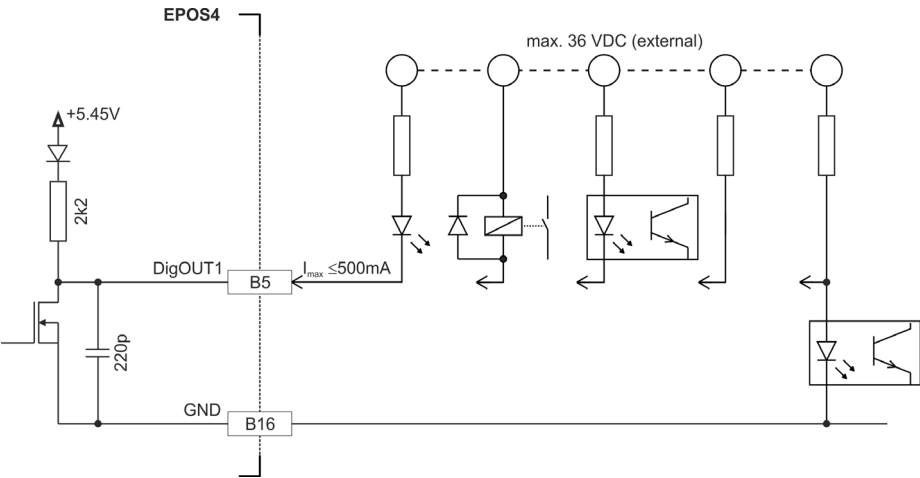
図 3-45 DigOUT1 “シンク” (DigOUT2 および Compact も同様)
