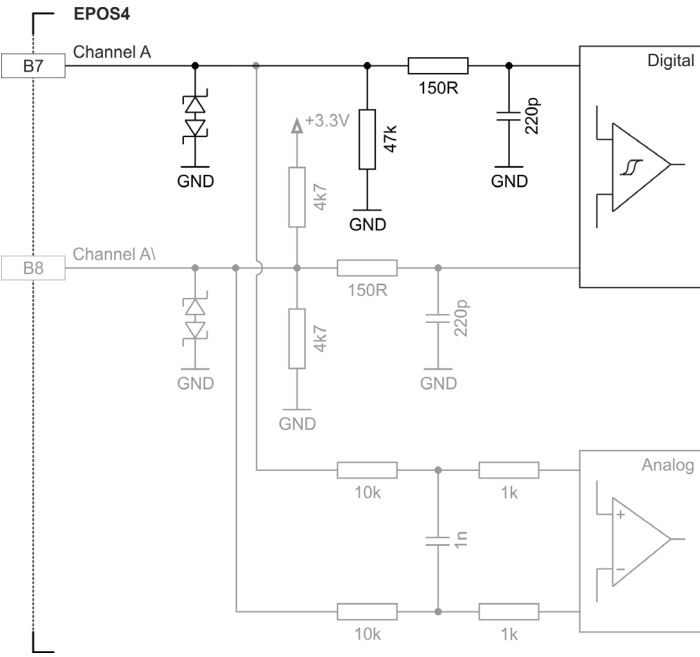
図 3-32 デジタル・インクリメンタル・エンコーダ入力回路 Ch A “単一端” (Ch B も同様)
