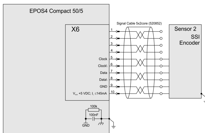
図 5-69 SSI アブソリュート・エンコーダ (Sensor 2)
