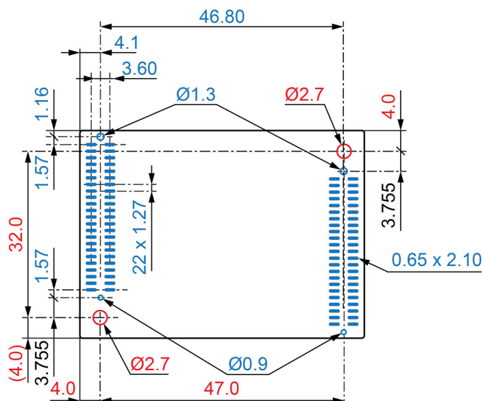
図 4-58 SMT フットプリント [mm] – 上から見た図
