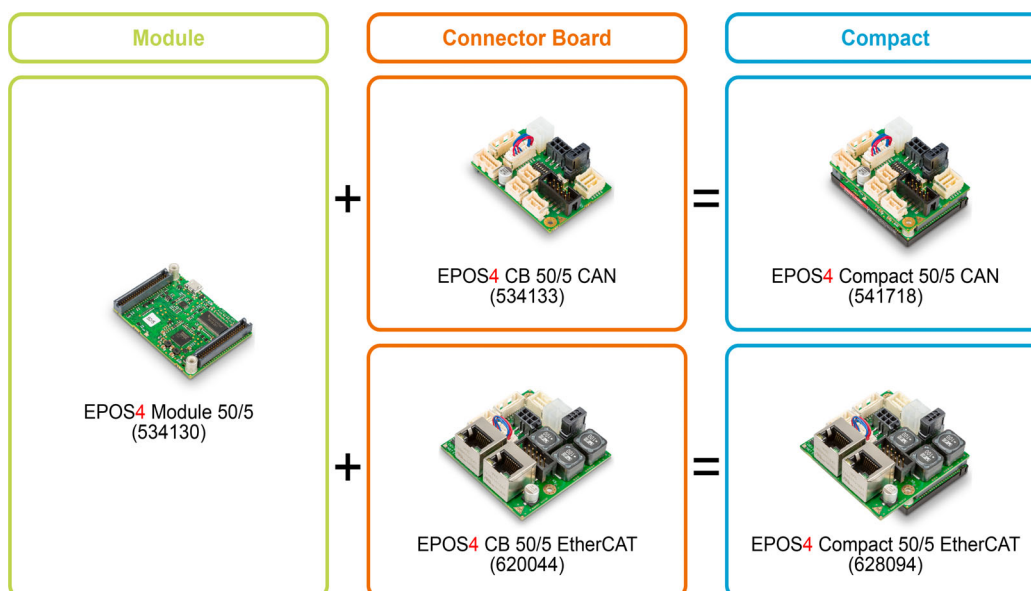
図 1-2 製品構成
