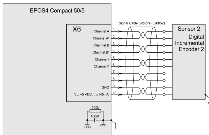
図 5-67 デジタル・インクリメンタル・エンコーダ 2 (Sensor 2)
