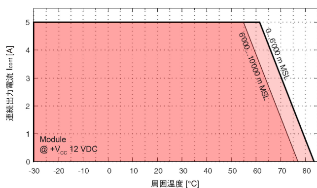
図 2-3 出力電流ディレーティング
