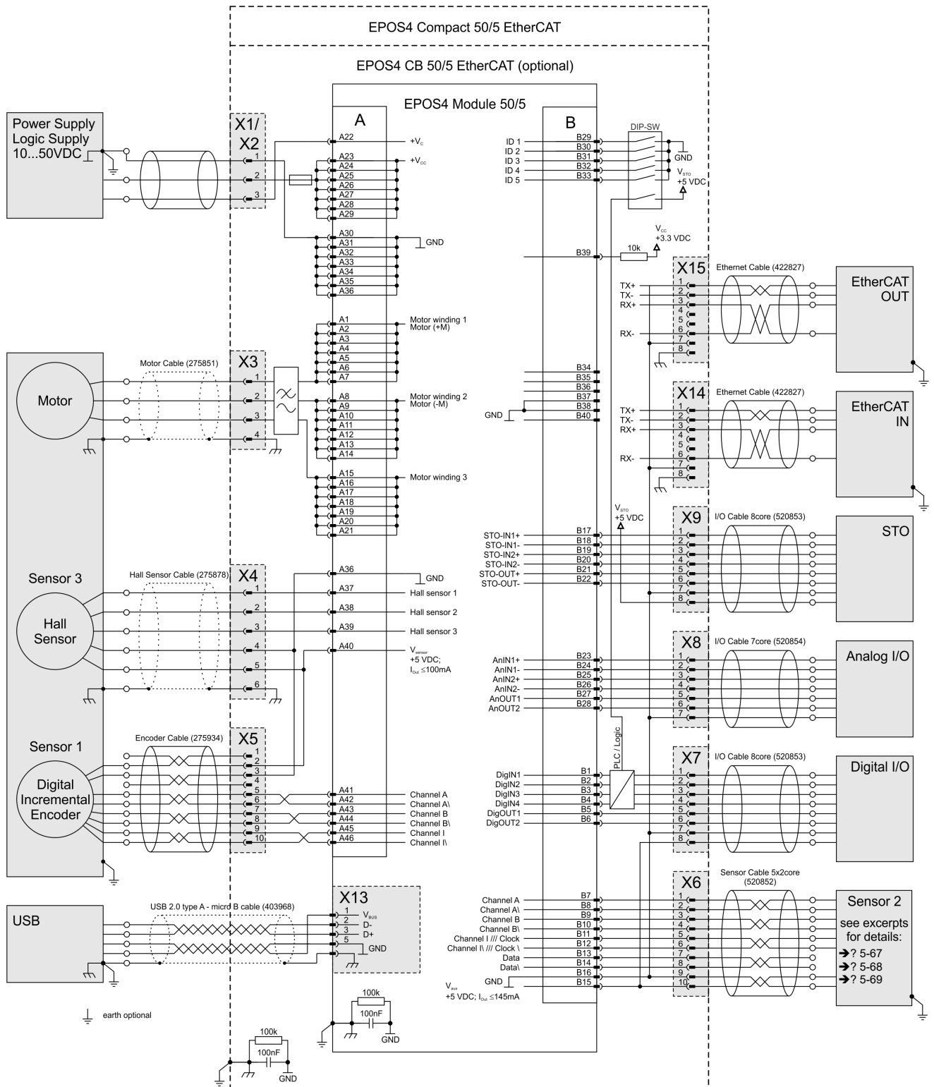
図 5-61 配線概要図 – Module & Compact EtherCAT
