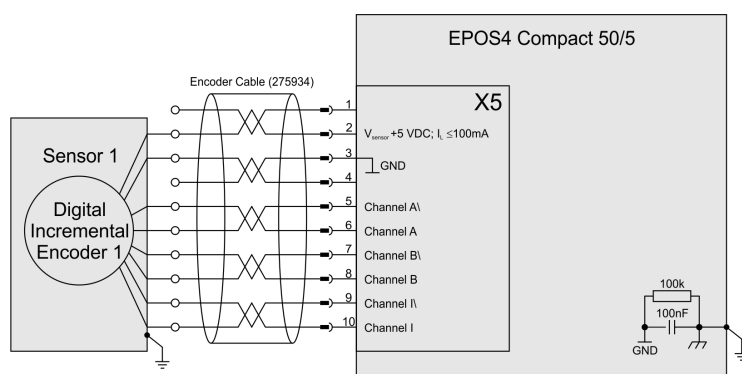
図 5-66 デジタル・インクリメンタル・エンコーダ 1 (Sensor 1)
