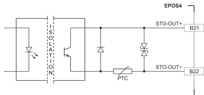
図 3-48 STO-OUT 回路
