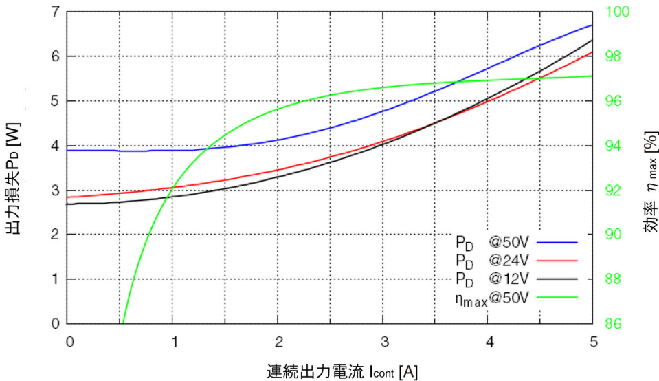
図 2-5 出力損失と効率 – EPOS4 Compact 50/5 EtherCAT
