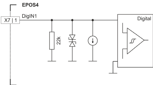
図 3-43 DigIN1 回路 (DigIN2...4 も同様) – Compact / PLC レベル設定
