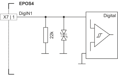
図 3-42 DigIN1 回路 (DigIN2...4 も同様) – Compact / ロジックレベル設定
