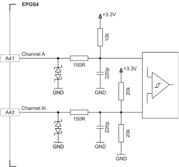
図 3-28 エンコーダ入力回路 Ch A “差動”（Ch B および Ch I も同様）
