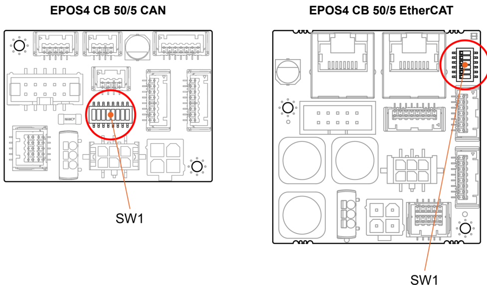
図 3-26 EPOS4 CB 50/5 CAN – DIP スイッチ SW1
