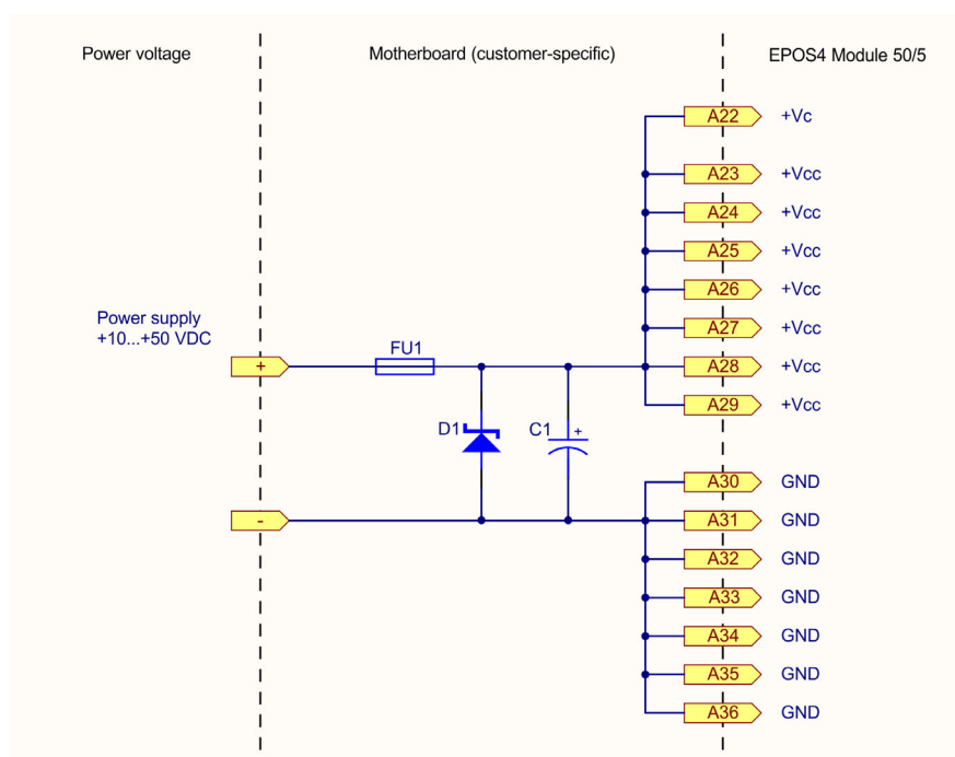
図 4-54 電源推奨配線
