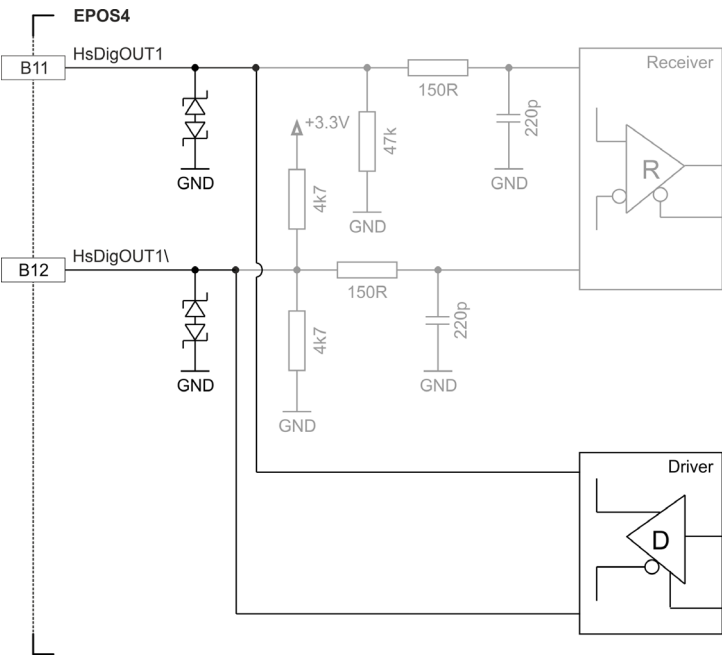
図 3-40 HsDigOUT1 出力回路
