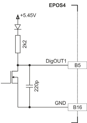
図 3-44 DigOUT1 回路 (DigOUT2 および Compact も同様)
