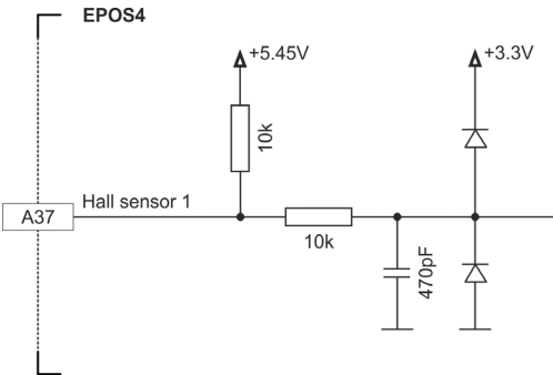
図 3-27 ホールセンサ 1 入力回路（ホールセンサ 2 および 3 も同様）
