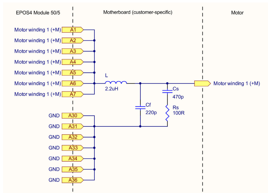
図 4-56 モータ巻線 1 推奨配線（巻線 2 および巻線 3 も同様）
