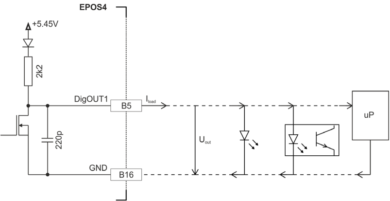
図 3-46 DigOUT1 “ソース” (DigOUT2 および Compact も同様)
