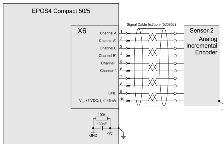
図 5-68 アナログ・インクリメンタル・エンコーダ (Sensor 2)
