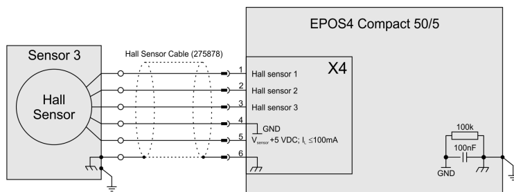
図 5-65 ホールセンサ (Sensor 3)
