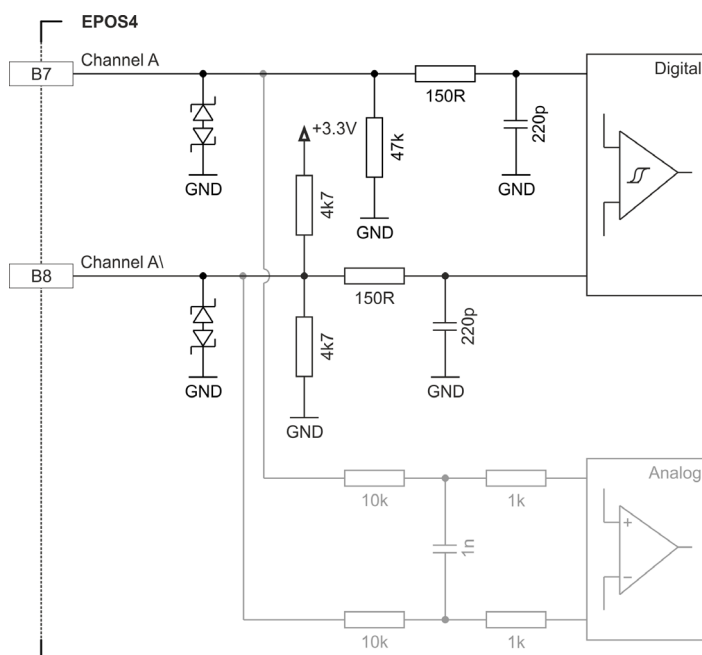
図 3-30 デジタル・インクリメンタル・エンコーダ入力回路 Ch A “差動” (Ch B も同様)
