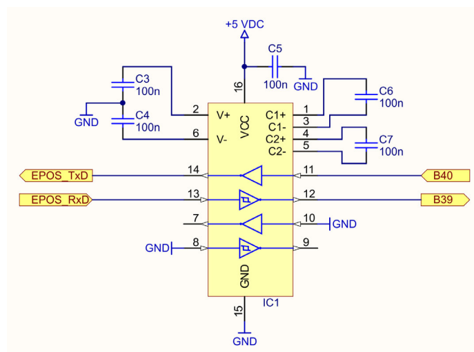
図 4-57 RS232 トランシーバ推奨配線
