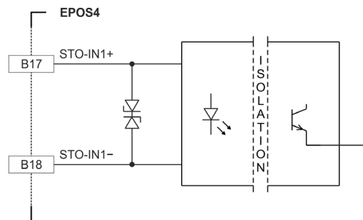
図 3-47 STO-IN1 回路 (STO-IN2 も同様)
