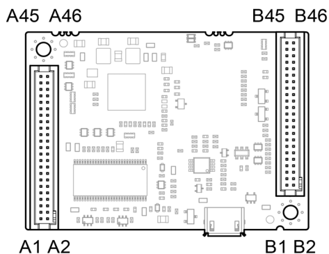
図 3-11 ピン配置
