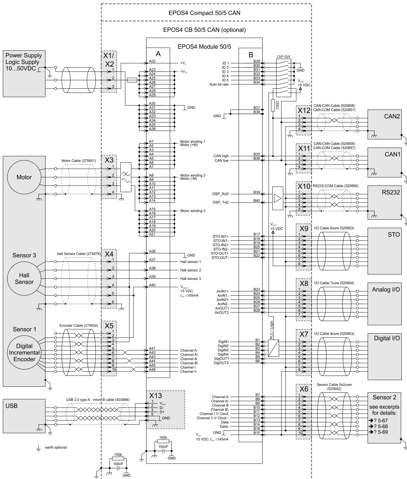
図 5-60 配線概要図 – Module & Compact CAN
