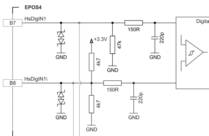
図 3-38 HsDigIN1 回路 “差動” (HsDigIN2...4 も同様)
