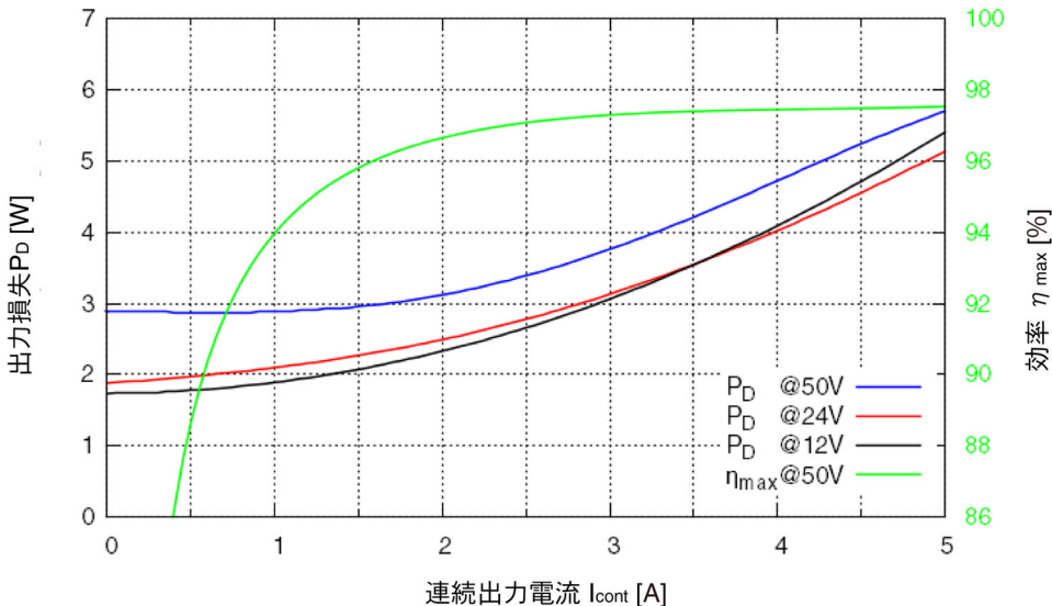
図 2-4 出力損失と効率 – EPOS4 Compact 50/5 CAN
