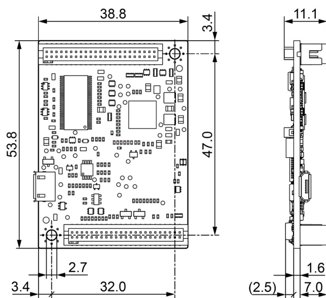
図 2-6 EPOS4 Module 50/5 – 外形寸法 [mm] (第一角法)
