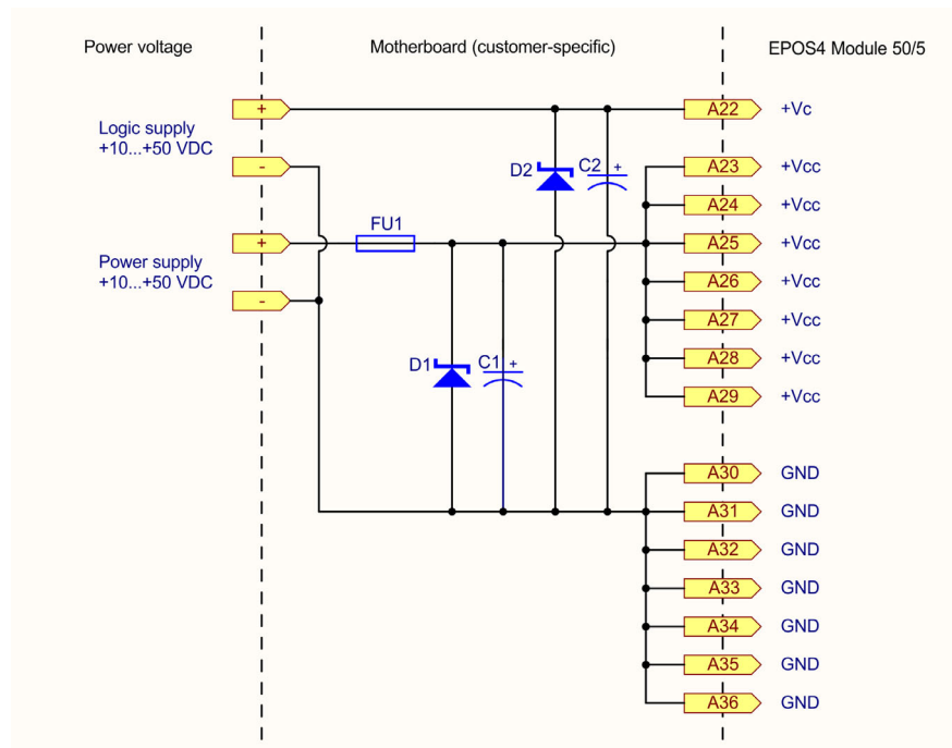
図 4-55 ロジック電源推奨配線
