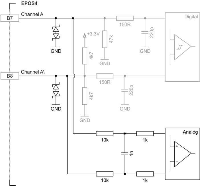
図 3-34 アナログ・インクリメンタル・エンコーダ入力回路 Ch A “差動”（Ch B も同様）
