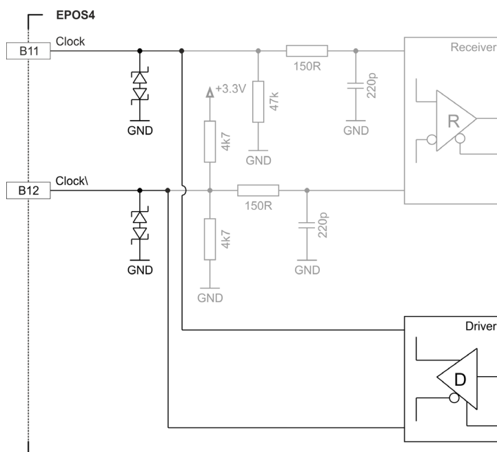
図 3-37 SSI アブソリュート・エンコーダ Clock 出力
