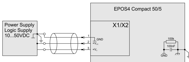
図 5-62 電源 & ロジック電源
