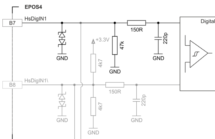
図 3-39 HsDigIN1 回路 “単一端” (HsDigIN2...4 も同様)
