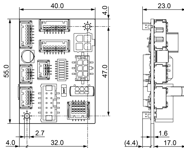
図 2-7 EPOS4 CB 50/5 CAN – 外形寸法 [mm] (第一角法)
