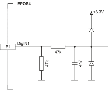
図 3-41 DigIN1 回路 (DigIN2...4 も同様) – Module
