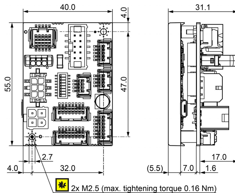
図 2-8 EPOS4 Compact 50/5 CAN – 外形寸法 [mm] (第一角法)
