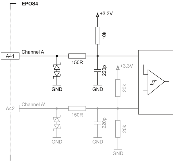
図 3-29 エンコーダ入力回路 Ch A “単一端”（Ch B および Ch I も同様）
