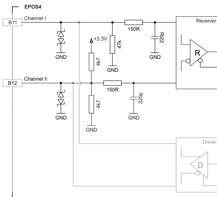
図 3-31 デジタル・インクリメンタル・エンコーダ入力回路 Ch I
