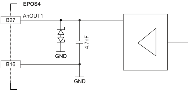
図 3-50 AnOUT1 回路（AnOUT2 も同様）
