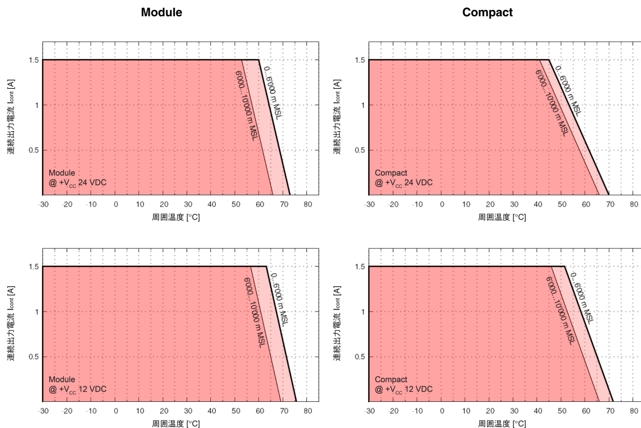
図 2-3 出力電流ディレーティング
