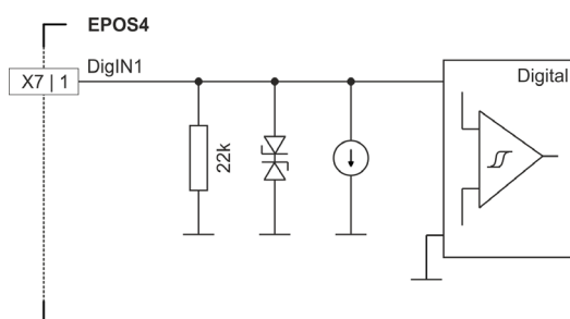
図 3-47 DigIN1 回路 (DigIN2...4 も同様) – Compact / PLC レベル設定
