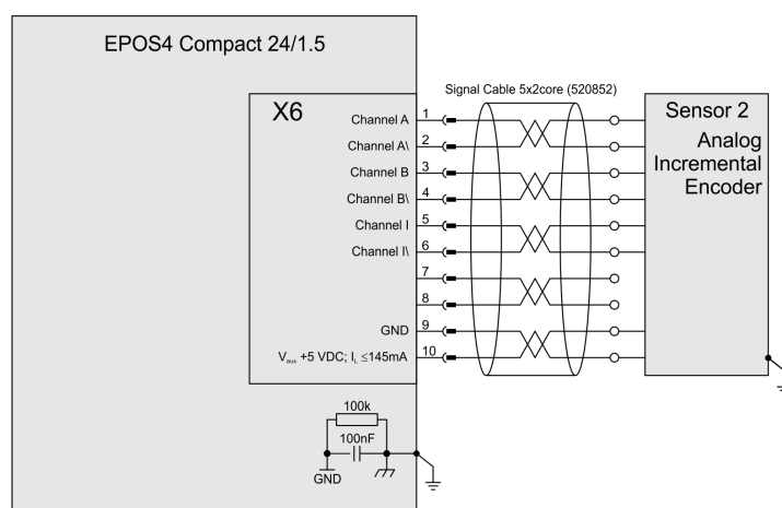
図 5-72 アナログ・インクリメンタル・エンコーダ (Sensor 2)
