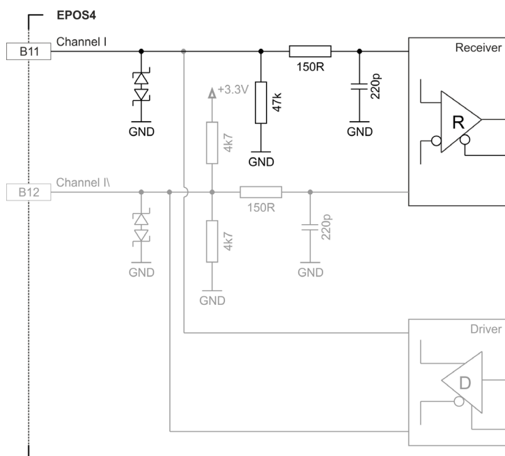
図 3-37 デジタル・インクリメンタル・エンコーダ入力回路 Ch I
