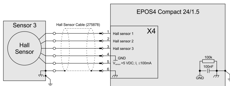
図 5-69 ホールセンサ (Sensor 3)
