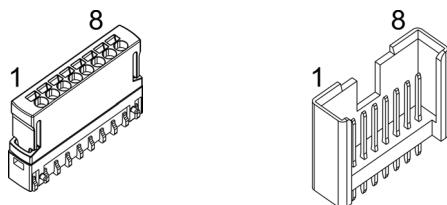
図 3-16 モータ / ホールセンサ・コンポコネクタ X3a/X4a (左) および X3b/X4b (右)
