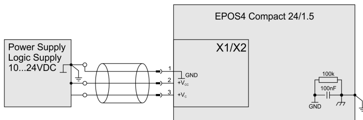
図 5-66 電源 & ロジック電源
