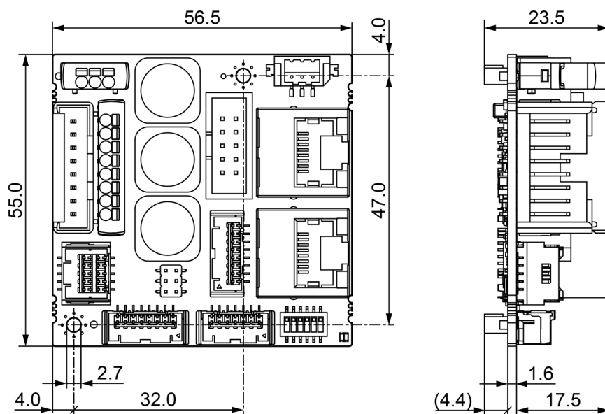
図 2-9 EPOS4 CB 24/1.5 EtherCAT – 外形寸法 [mm] (第一角法)
