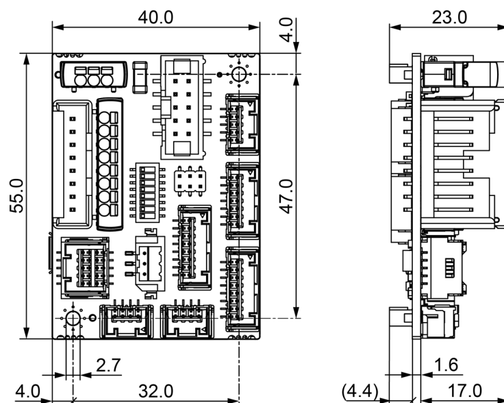
図 2-7 EPOS4 CB 24/1.5 CAN – 外形寸法 [mm] (第一角法)
