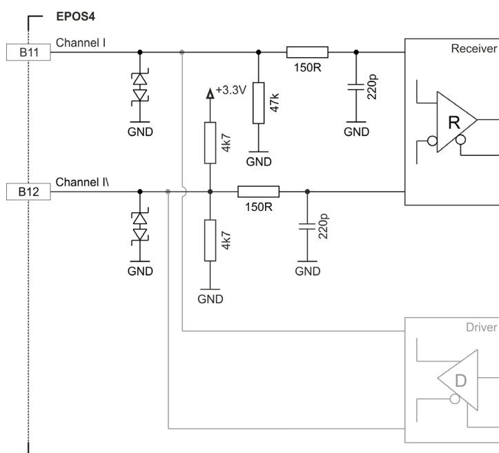
図 3-35 デジタル・インクリメンタル・エンコーダ入力回路 Ch I
