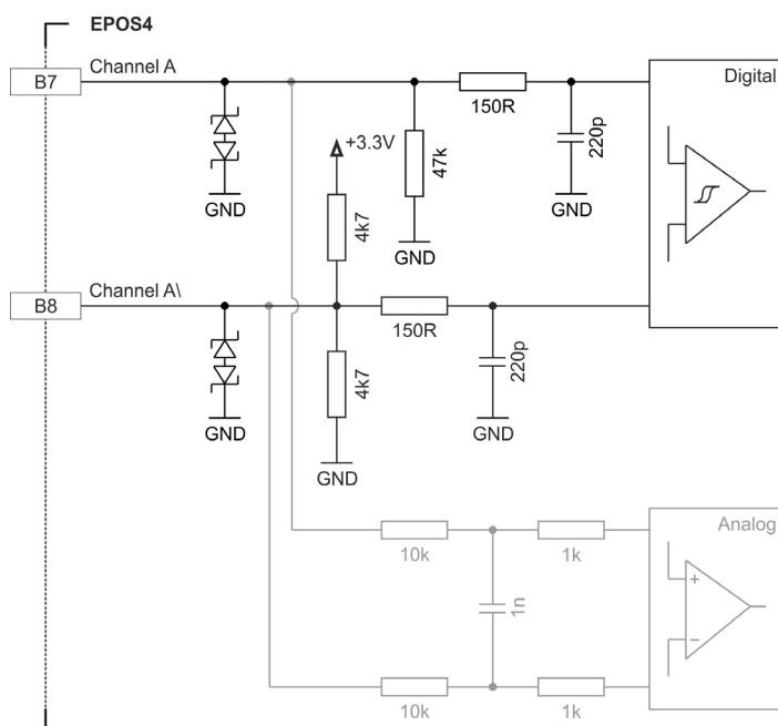
図 3-34 デジタル・インクリメンタル・エンコーダ入力回路 Ch A “差動” (Ch B も同様)
