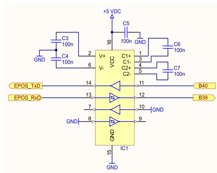
図 4-61 RS232 トランシーバ推奨配線
