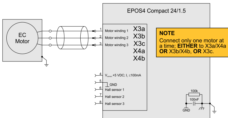
図 5-68 EC (BLDC) モータ
