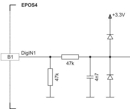
図 3-45 DigIN1 回路 (DigIN2...4 も同様) – Module
