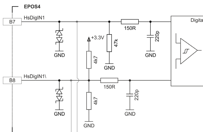
図 3-42 HsDigIN1 回路 “差動” (HsDigIN2...4 も同様)
