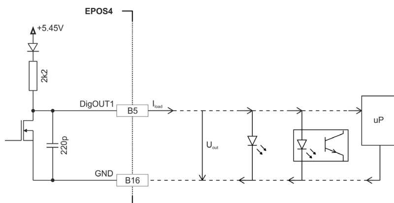
図 3-50 DigOUT1 “ソース” (DigOUT2 および Compact も同様)
