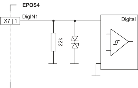
図 3-46 DigIN1 回路 (DigIN2...4 も同様) – Compact / ロジックレベル設定
