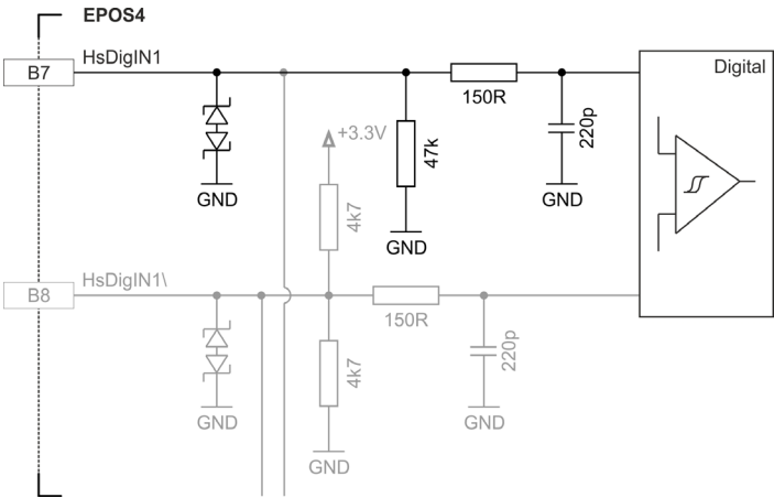
図 3-43 HsDigIN1 回路 “単一端” (HsDigIN2...4 も同様)
