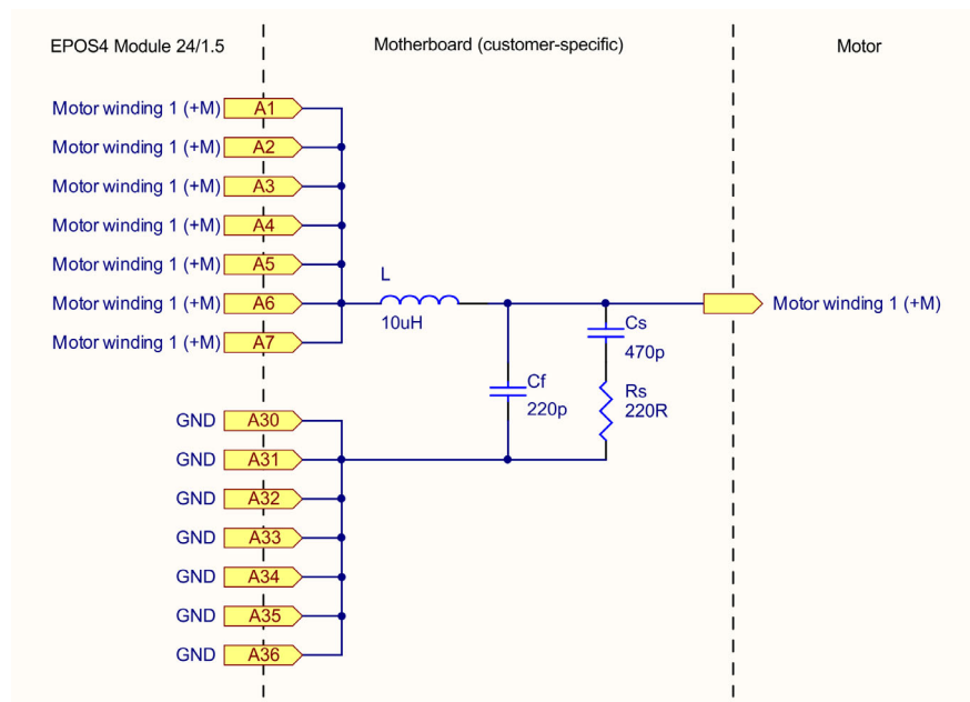
図 4-60 モータ巻線 1 推奨配線（巻線 2 および巻線 3 も同様）
