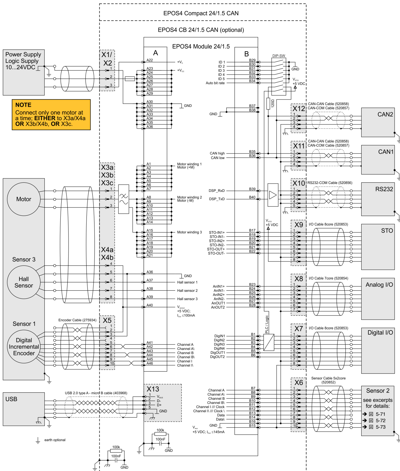
図 5-64 配線概要図 – Module & Compact CAN
