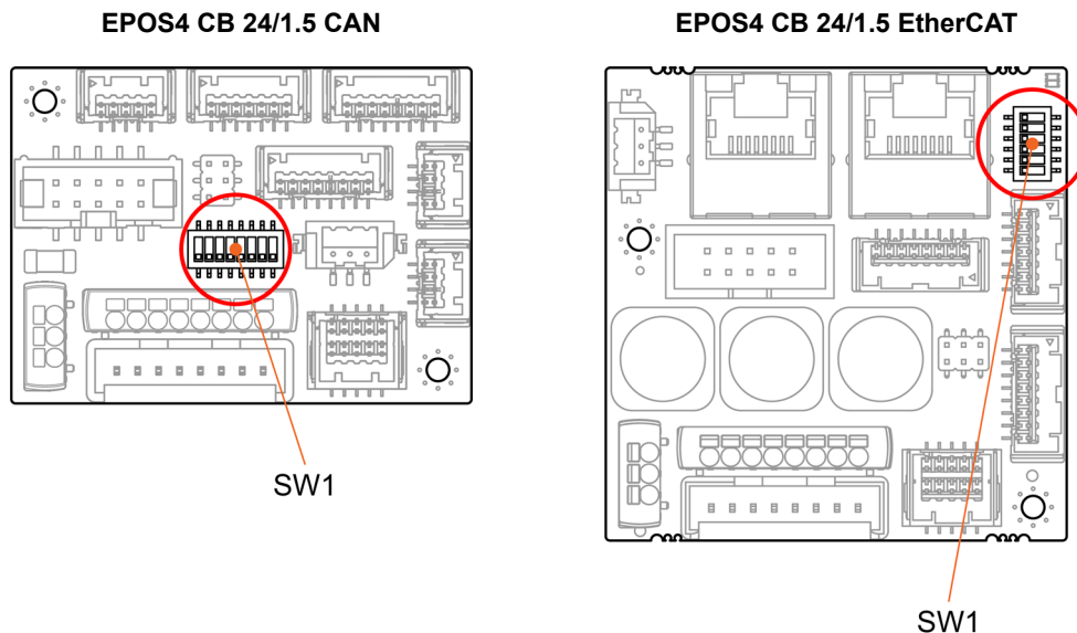
図 3-29 EPOS4 CB 24/1.5 CAN – DIP スイッチ SW1
