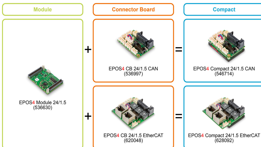
図 1-2 製品構成
