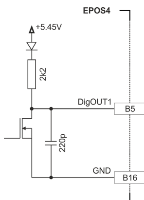
図 3-48 DigOUT1 回路 (DigOUT2 および Compact も同様)
