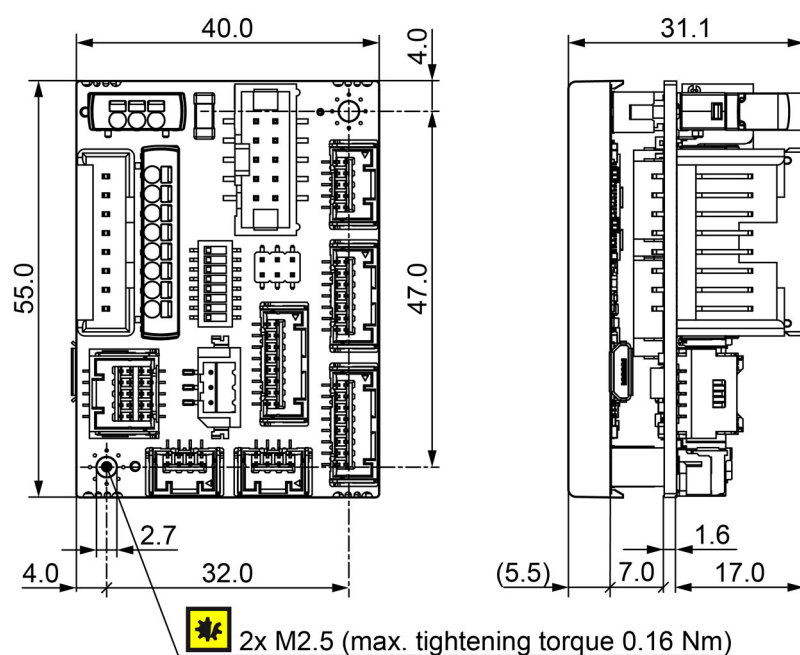
図 2-8 EPOS4 Compact 24/1.5 CAN – 外形寸法 [mm] (第一角法)
