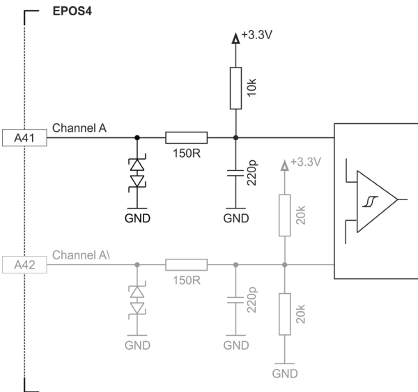
図 3-33 エンコーダ入力回路 Ch A “単一端”（Ch B および Ch I も同様）
