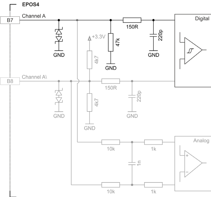
図 3-36 デジタル・インクリメンタル・エンコーダ入力回路 Ch A “単一端” (Ch B も同様)
