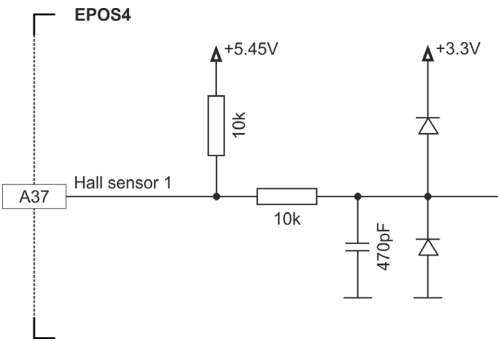
図 3-31 ホールセンサ 1 入力回路 (ホールセンサ 2 および 3 も同様)
