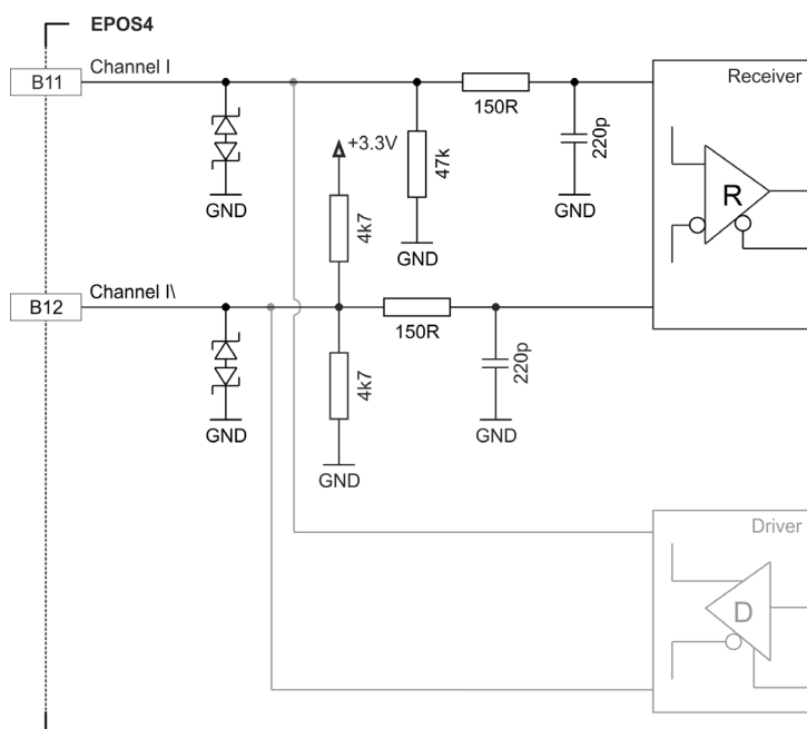
図 3-39 アナログ・インクリメンタル・エンコーダ入力回路 Ch I
