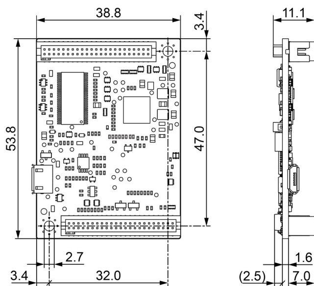
図 2-6 EPOS4 Module 24/1.5 – 外形寸法 [mm] (第一角法)
