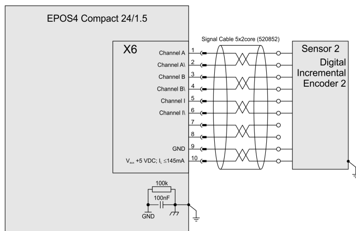
図 5-71 デジタル・インクリメンタル・エンコーダ 2 (Sensor 2)
