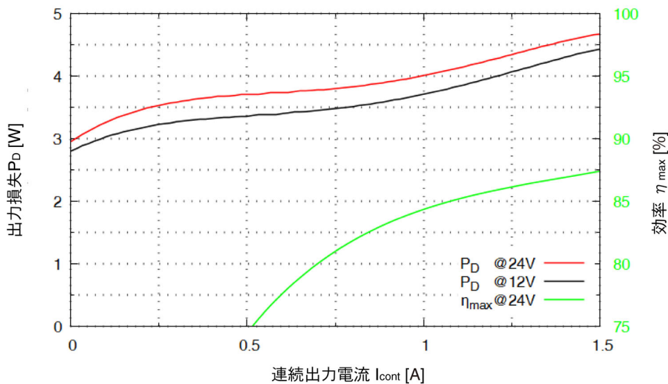
図 2-5 出力損失と効率 – EPOS4 Compact 24/1.5 EtherCAT
