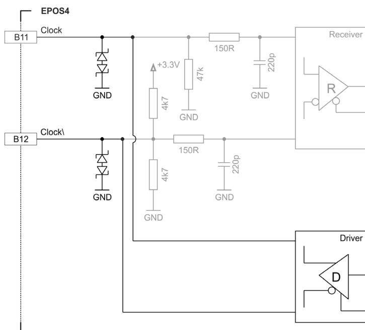
図 3-41 SSI アブソリュート・エンコーダ Clock 出力
