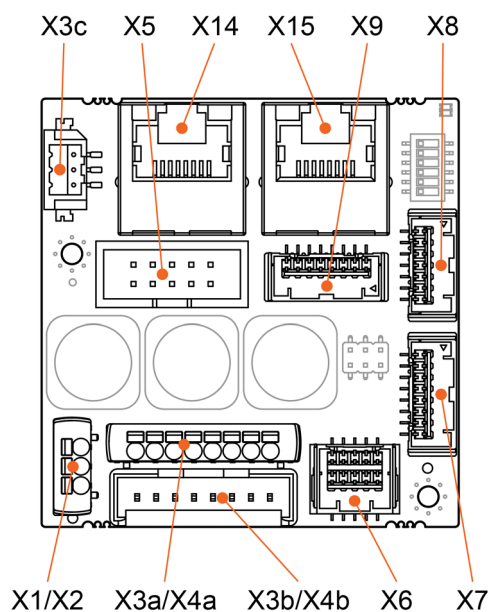
図 3-14 EPOS4 CB 24/1.5 – 接続
