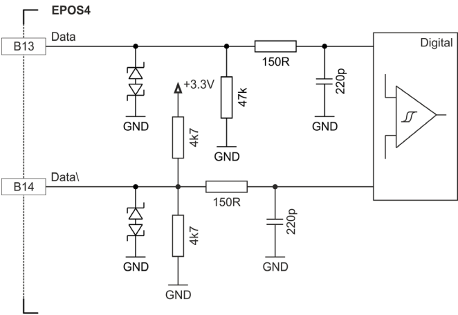
図 3-40 SSI アブソリュート・エンコーダ Data 入力
