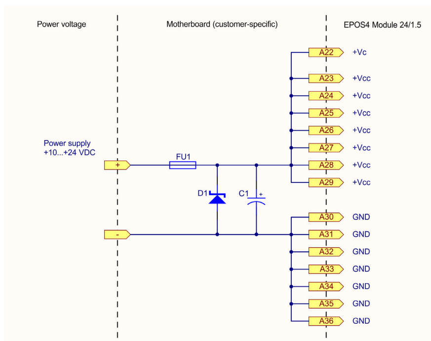
図 4-58 電源推奨配線
