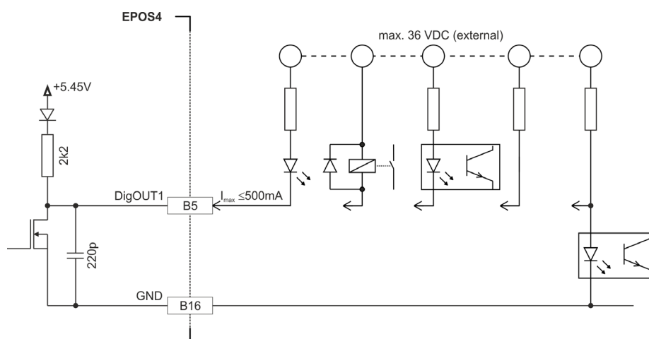
図 3-49 DigOUT1 “シンク” (DigOUT2 および Compact も同様)
