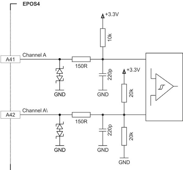
図 3-32 エンコーダ入力回路 Ch A “差動”（Ch B および Ch I も同様）
