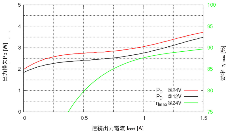
図 2-4 出力損失と効率 – EPOS4 Compact 24/1.5 CAN
