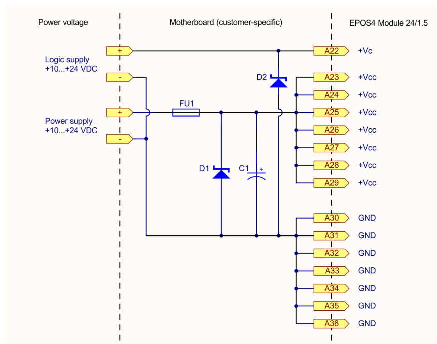
図 4-59 ロジック電源推奨配線
