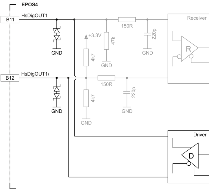
図 3-44 HsDigOUT1 出力回路
