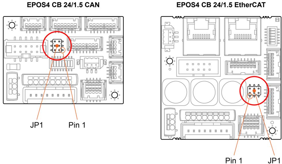
図 3-30 EPOS4 CB 24/1.5 – ジャンパ JP1
