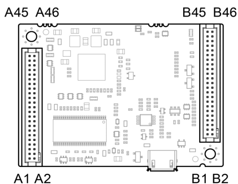
図 3-11 ピン配置
