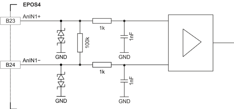
図 3-53 AnIN1 回路（AnIN2 も同様）
