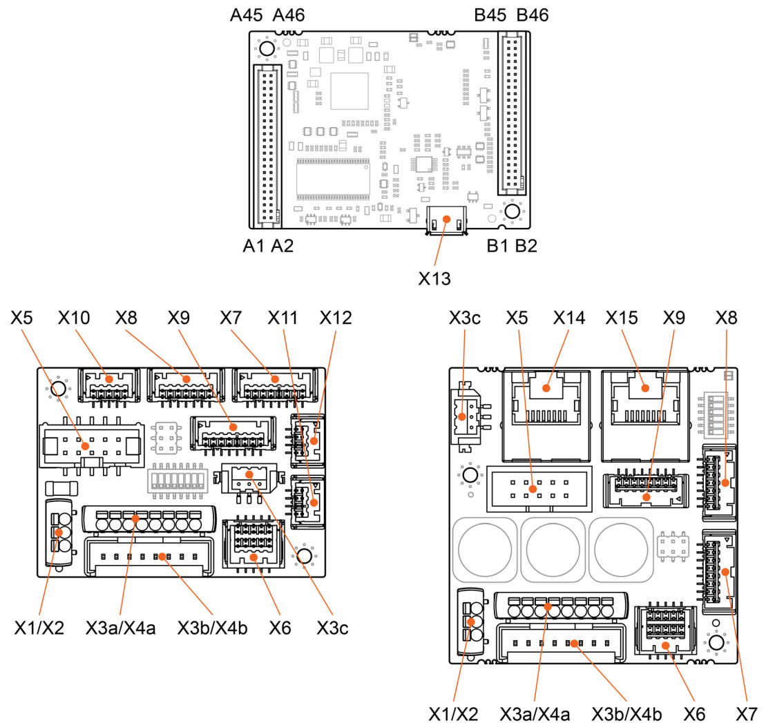
図 5-63 インターフェイス – 名称と取り付け位置
