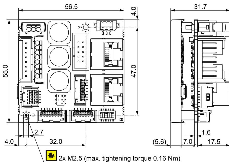
図 2-10 EPOS4 Compact 24/1.5 EtherCAT – 外形寸法 [mm] (第一角法)
