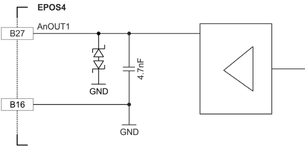
図 3-54 AnOUT1 回路（AnOUT2 も同様）
