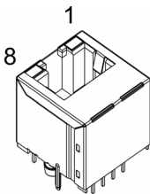
図 3-25 EtherCAT IN & EtherCAT OUT コネクタ X14 & X15
