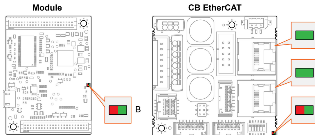
図 3-57 状態表示 LED
