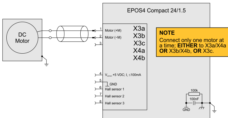
図 5-67 DC モータ
