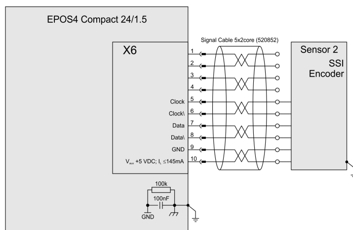
図 5-73 SSI アブソリュート・エンコーダ (Sensor 2)
