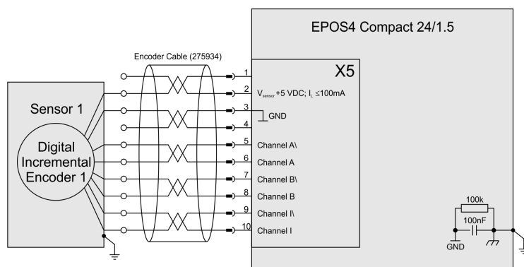
図 5-70 デジタル・インクリメンタル・エンコーダ 1 (Sensor 1)
