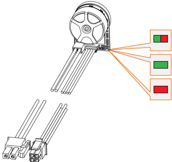
図 3-9 状態表示 LED
