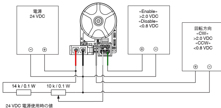
図 4-12 24 VDC 電源使用時の値 回転数設定：ポテンショメータ、「Enable」および回転方向：外部電源使用
