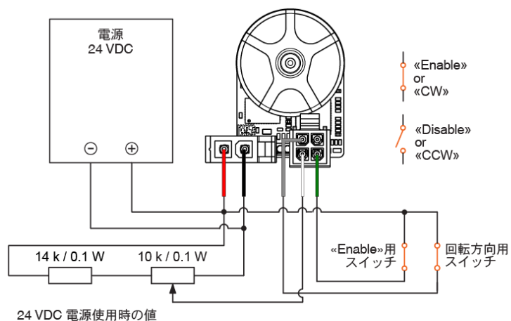
図 4-13 24 VDC 電源使用時の値 回転数設定：ポテンショメータ、「Enable」および回転方向：スイッチ（ポテンシャルフリー接点）使用
