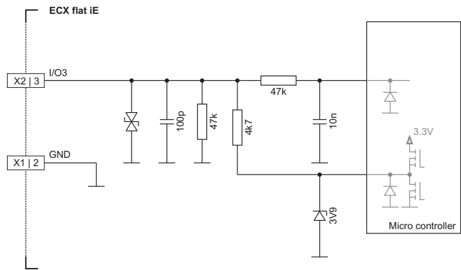
図 3-8 I/O 3, I/O 4 | 内部回路
